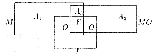
Рис.1. Классификация реальных объектов. I – идеи, объекты, представленные в индивидуальном сознании образами; M – материя; MO – материальные оболочки – торсионные поля, сопутствующие идеям; F – фантомы – устойчивые MO ; O – пустые множества; A_1 – материя о которой ничего не известно; A_2 – MO , сопутствующие идеям нематериальных объектов; A_3 – неустойчивые MO идей материальных объектов.
