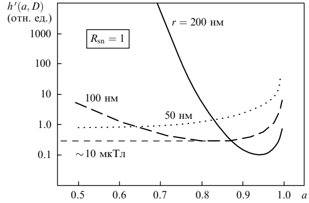
Рис.2. Предельная чувствительность магнитосом разных размеров к переменному МП. Уровень 10 мкТл рассчитан для H = H_{geo} .
